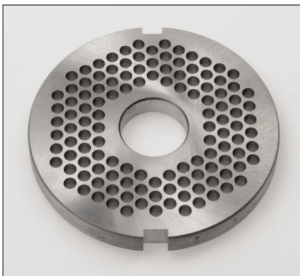
Lochscheibe D114 codiert (2 gleich grosse Nuten)
