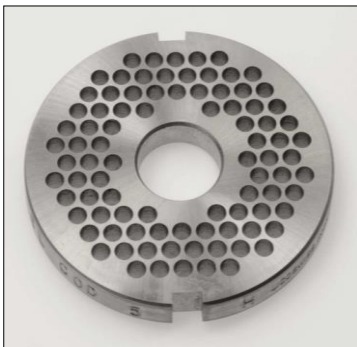
Lochscheibe H82 codiert (2 gleich grosse Nuten)
